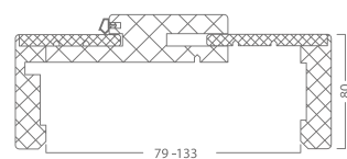
Моноблок тип МБ 79-133 Monoblock type MB 79-133
