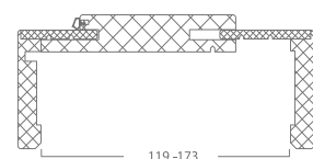
Моноблок тип МБ 119-173 Monoblock type MB 119-173
