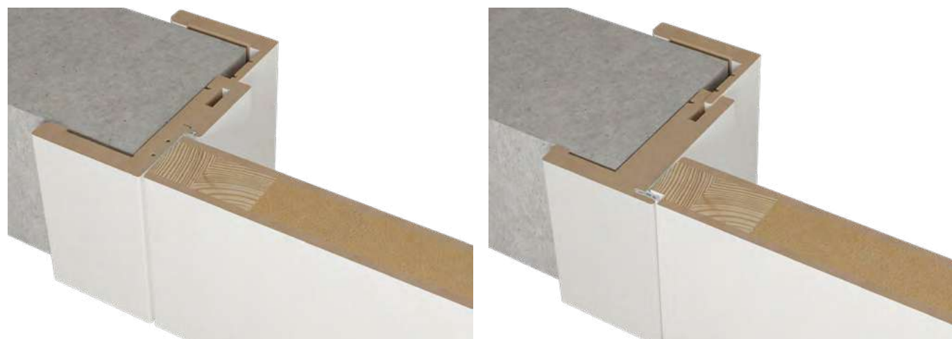
Стойка дверной коробки моноблок тип /МБ 79-133 (четв. 43 / 49). Наличник фанерованный 80/55. Door jamb monoblock type MB 73-133 (groove 43 / 49). Veneered 80/55 casing.
