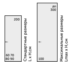
Короб А45
