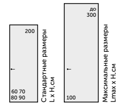
Короб А45
